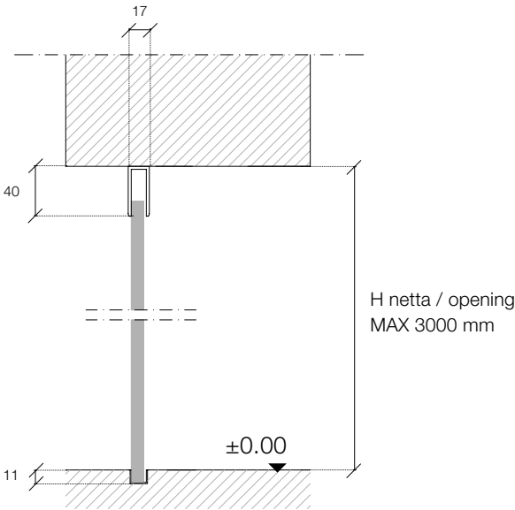
Profilo Orizzontale / A soffitto Horizontal Profile / Ceiling-mounted
