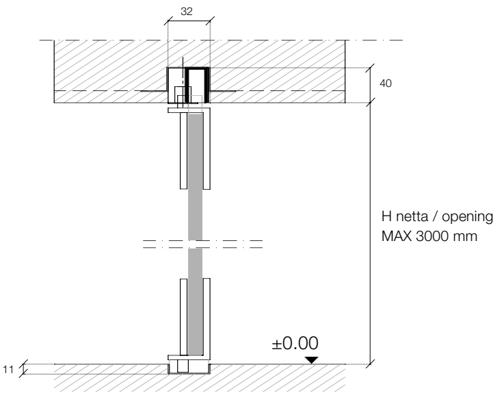
Profilo Orizzontale / A incasso Horizontal Profile / Recessed
