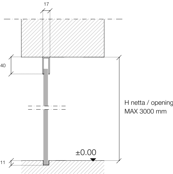
Profilo Orizzontale / A soffitto Horizontal Profile / Ceiling-mounted
