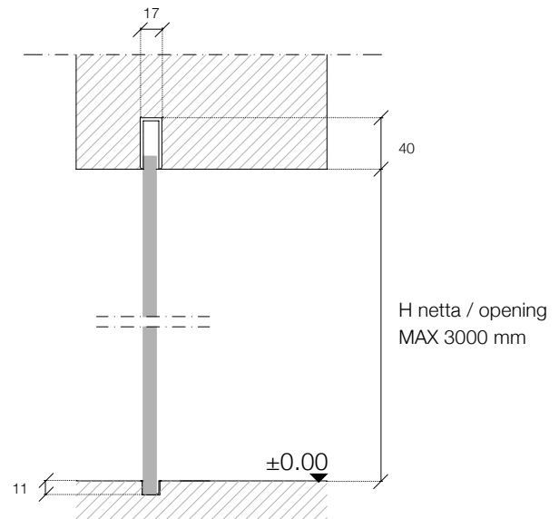
Profilo Orizzontale / A incasso Horizontal Profile / Recessed
